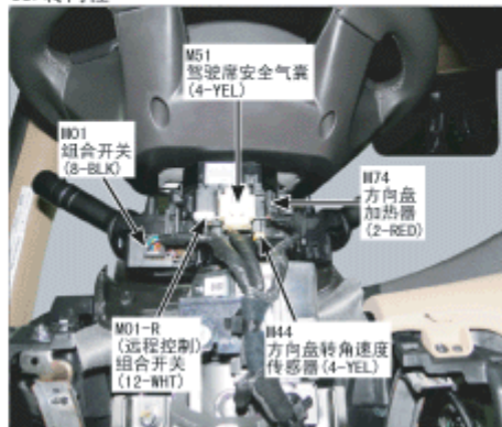
68. 转向柱
